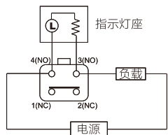
不动作时亮灯，常开触点正常打开时
