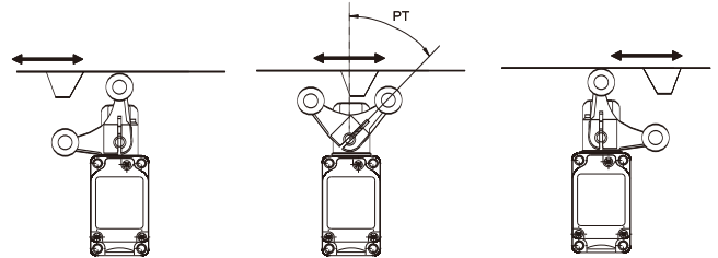
NC导通
