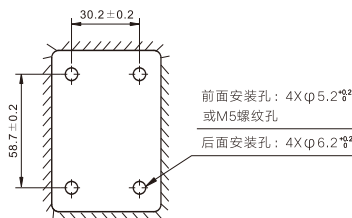
注：根据前面或后面安装方式选择开孔
