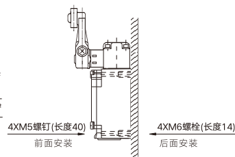
注：以上安装螺钉随产品附件提供
