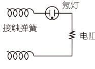
氖灯
