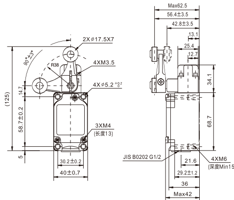
KXL-717 KXL-737 KXL-727 KXL-747 叉形滚轮手柄型
