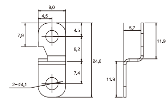
上图所示短路端子使用时能做单极双投型1C触点
