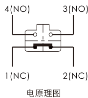
电原理图
