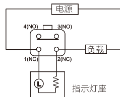
动作时亮灯，常闭触点动作打开时
