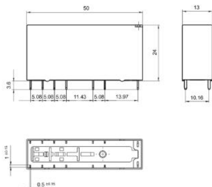
外形图(单位:毫米)
