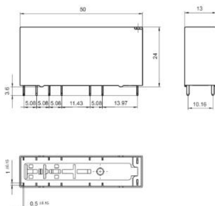
外形图(单位:毫米)
