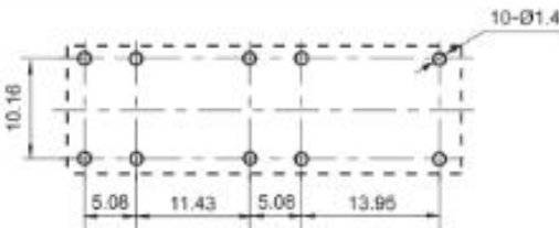
PCB 配置图(仰视图)
