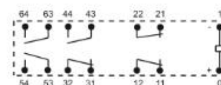
PCB 配置图(仰视图)
