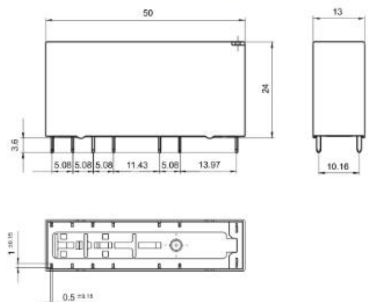
外形图(单位:毫米)
