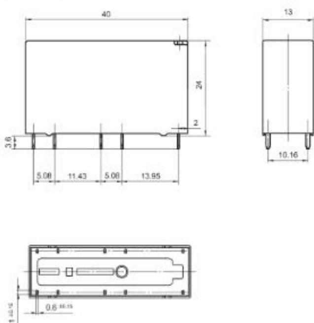
外形图(单位:毫米)
