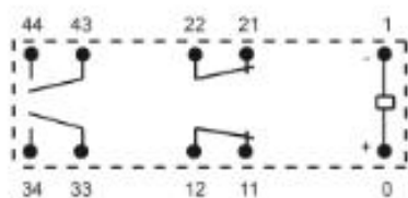
PCB 配置图(仰视图)
