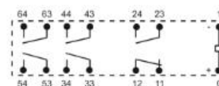
PCB 配置图(仰视图)
