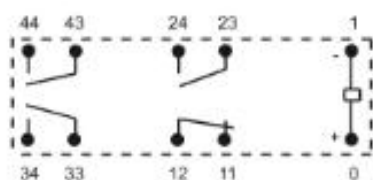
接线图 仰视图
