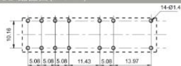
PCB 配置图(仰视图)
