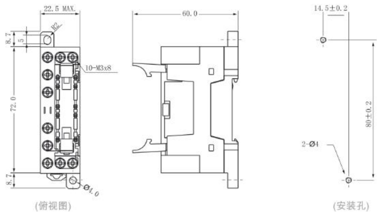
外形图
