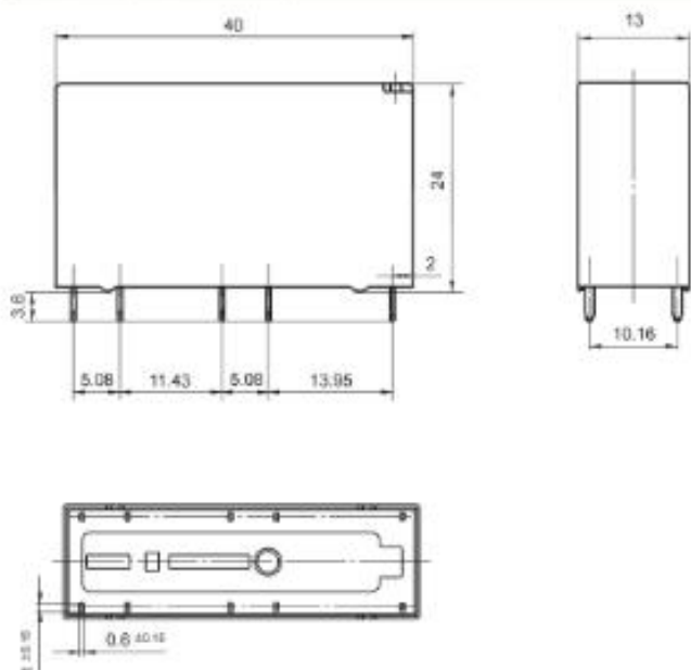
外形图(单位:毫米)
